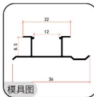
模具图
