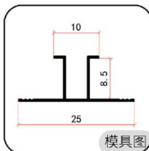
模具图
